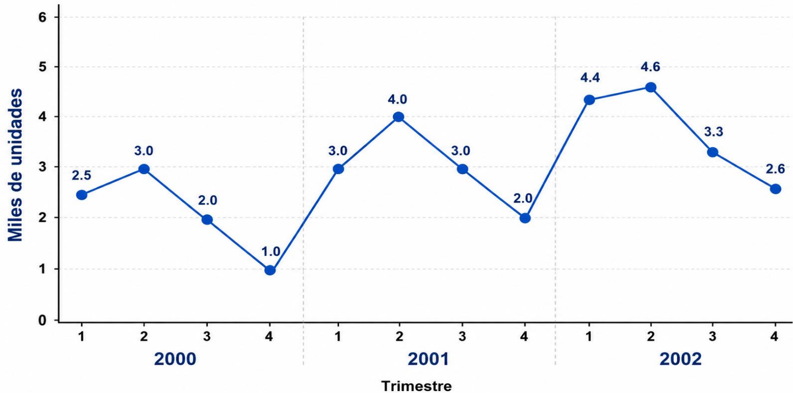
Ventas trimestrales de unidades (en miles)
