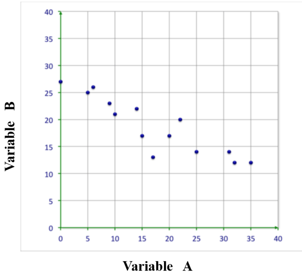
Gráfico de dispersión
