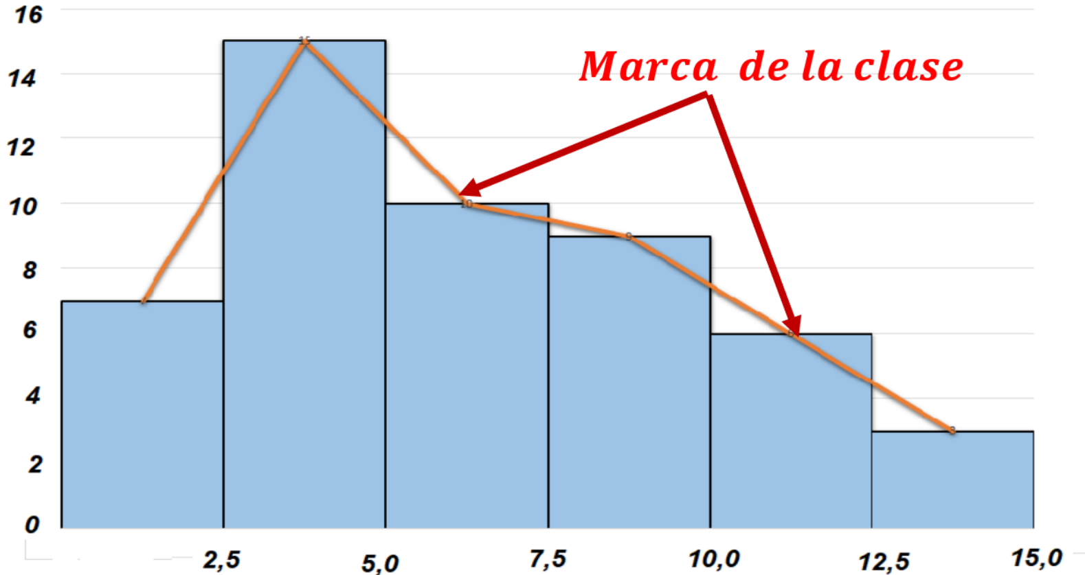
Histograma con polígono de frecuencias
