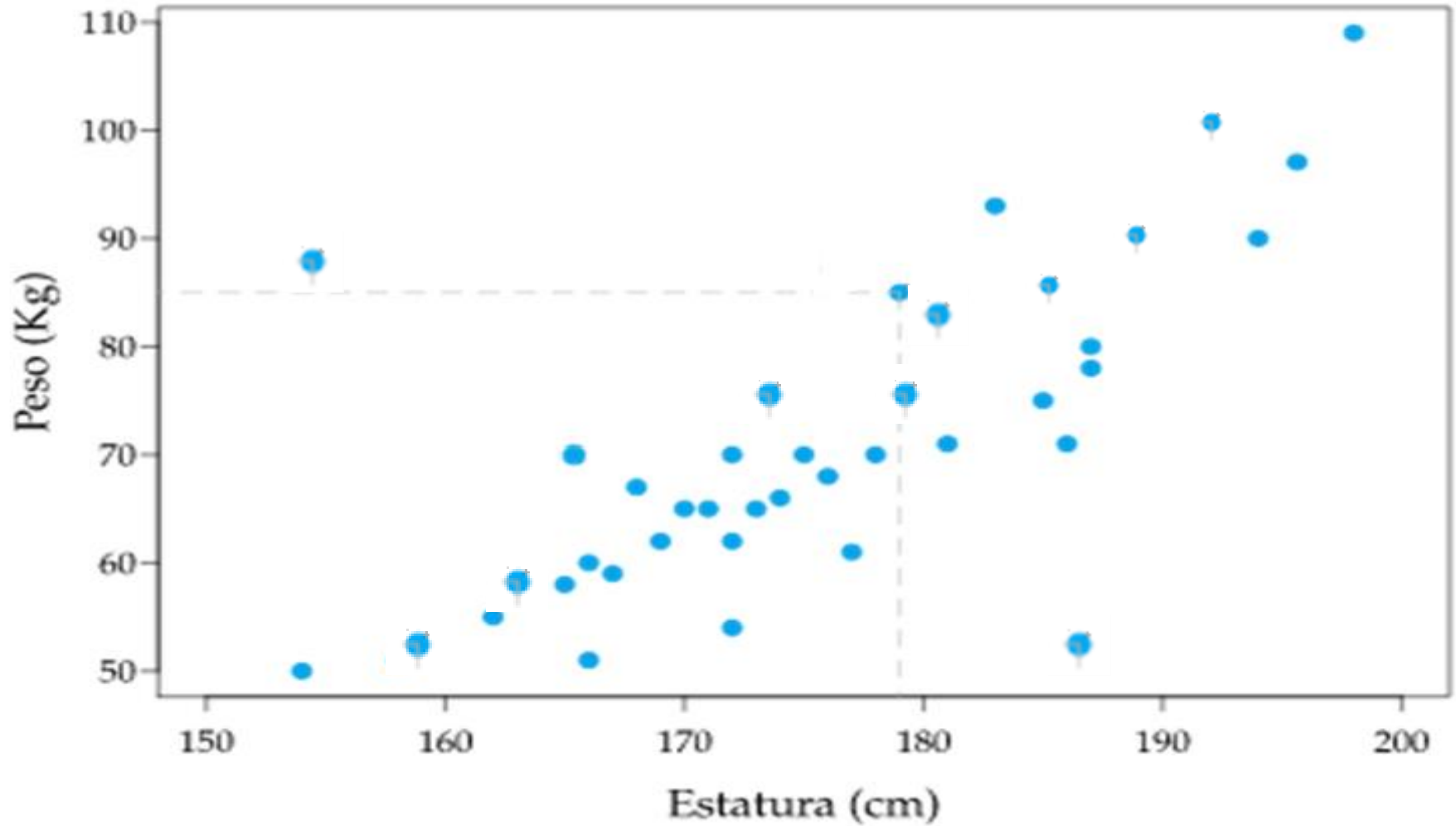
Diagrama de dispersión de estaturas y pesos
