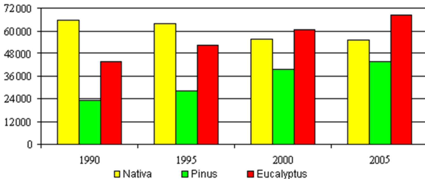
Gráfica de barras agrupadas
